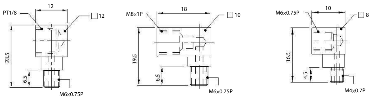
油管接頭型式
