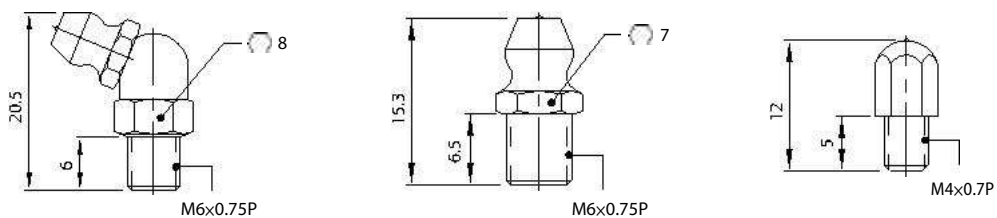
油嘴型式
